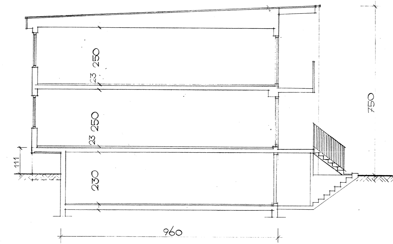
SEKTION A-A
