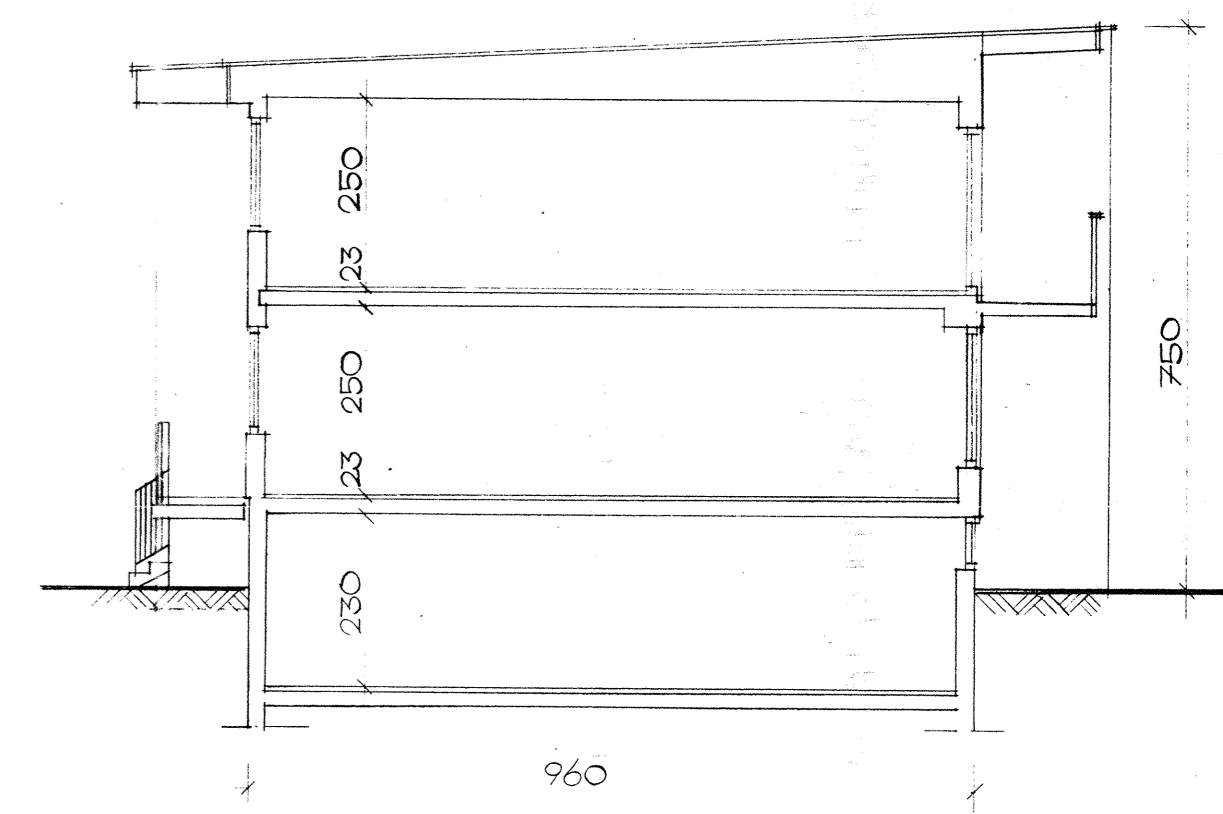
SEKTION B-B
